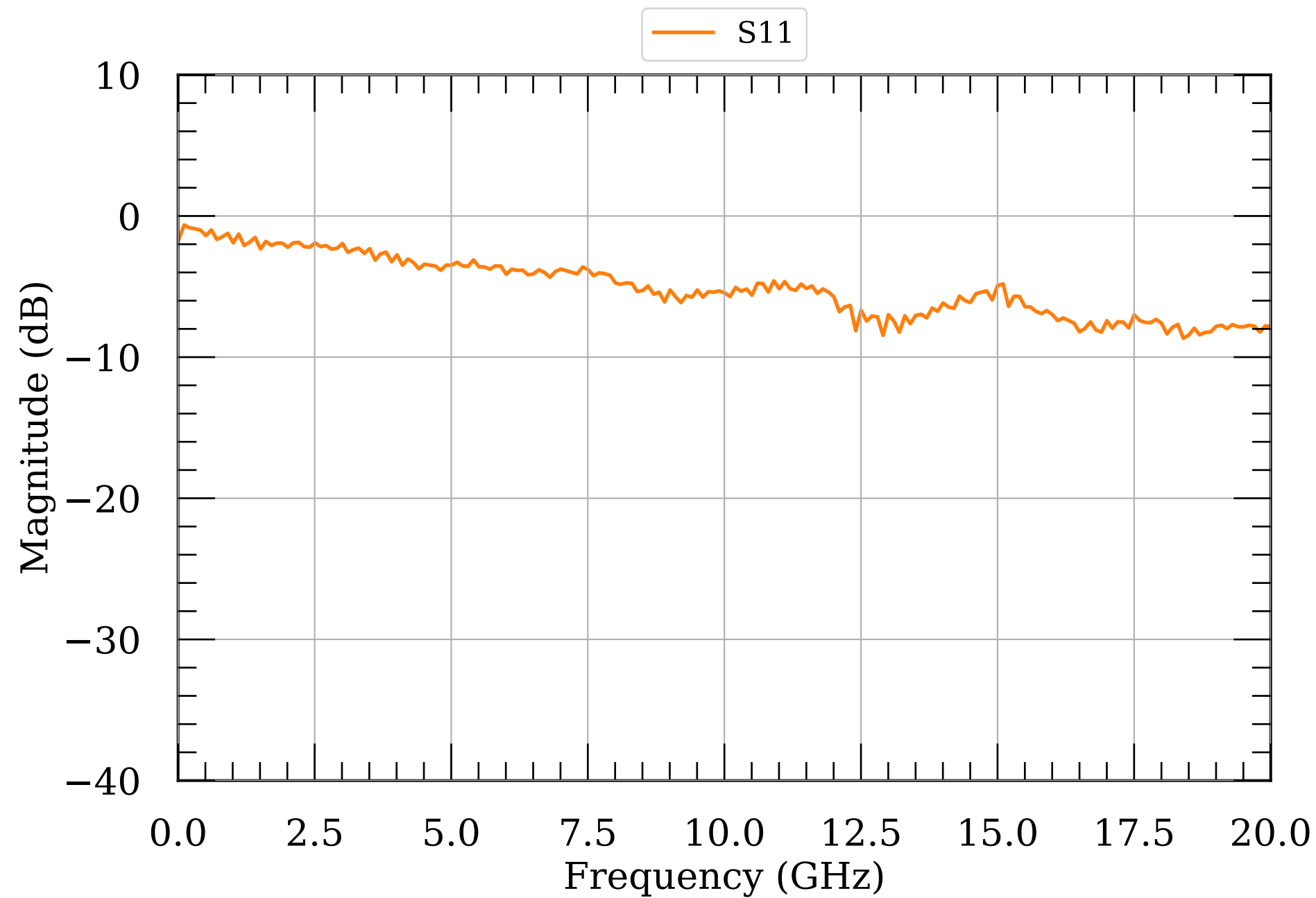
LNA S-params module010
